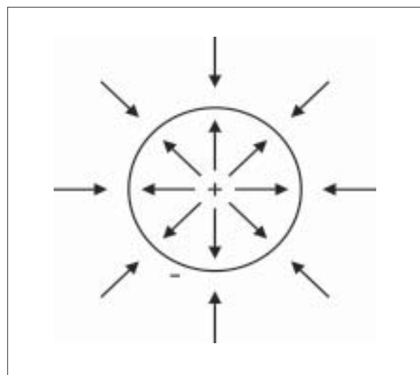
Bild 1: Meyl'scher Potenzialwirbel
