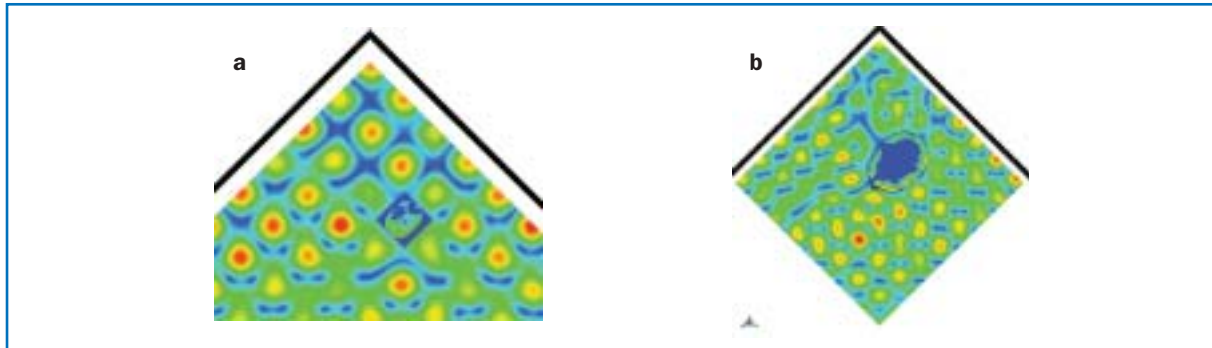
Bild 6: SAR-Verteilung im Kopf, a) bei 900 MHz, b) bei 2,45 GHz
