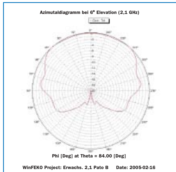
Bild 13: Azimutale Richtungscharakteristik des am Oberarm befestigten Dosimeters bei 2,1 GHz, Elevation 6 Grad
