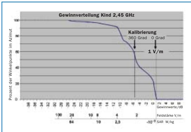
Bild 10: Gewinnverteilung in Abhängigkeit vom Azimutwinkel (Beispiel Kind, 2,45 GHz)
