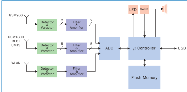
Bild 9: Schaltschema des Dosimeters
