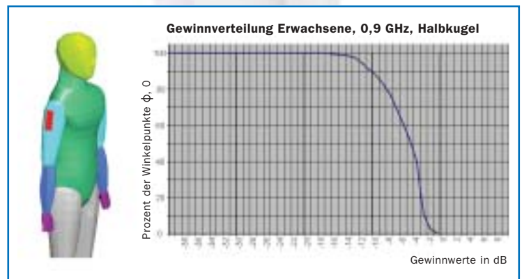
Bild 7: Berechnete Bedeckung der oberen Halbkugel (5275 Werte, auf maximalen Gewinn normiert)
