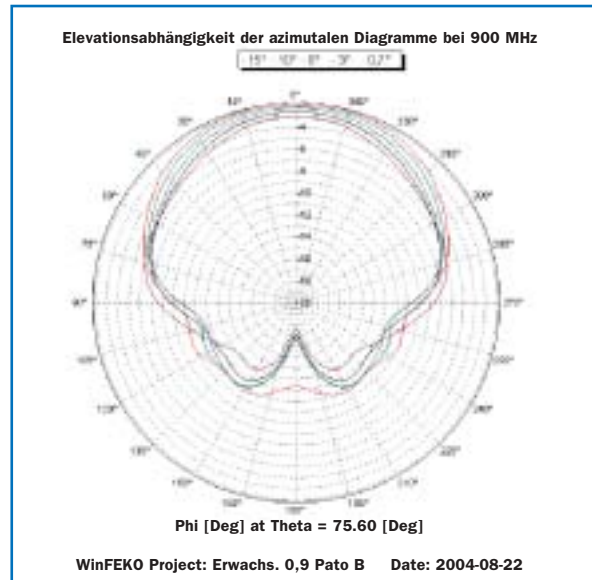
Bild 12: Azimutale Richtungscharakteristik des am Oberarm befestigten Dosimeters bei 900 MHz, Elevation variabel ( 15, 10, 6, 3, 0,7 Grad)
