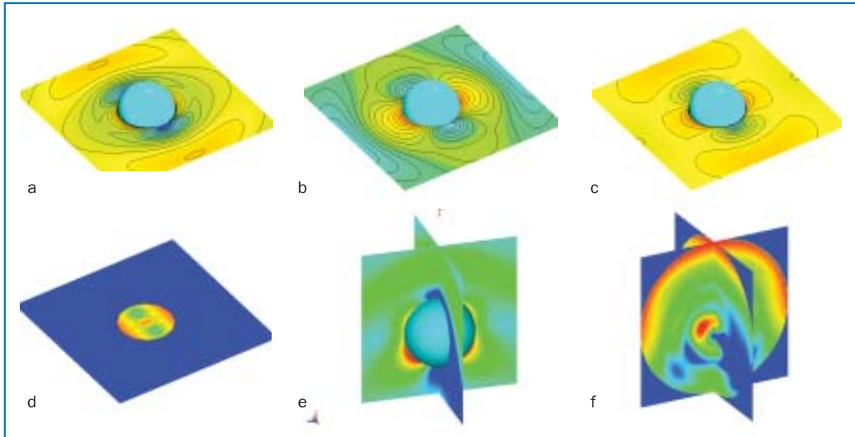
Bild 3: Feldverteilungen bei einer verlustbehafteten dielektrischen Kugel (ebene Welle)
