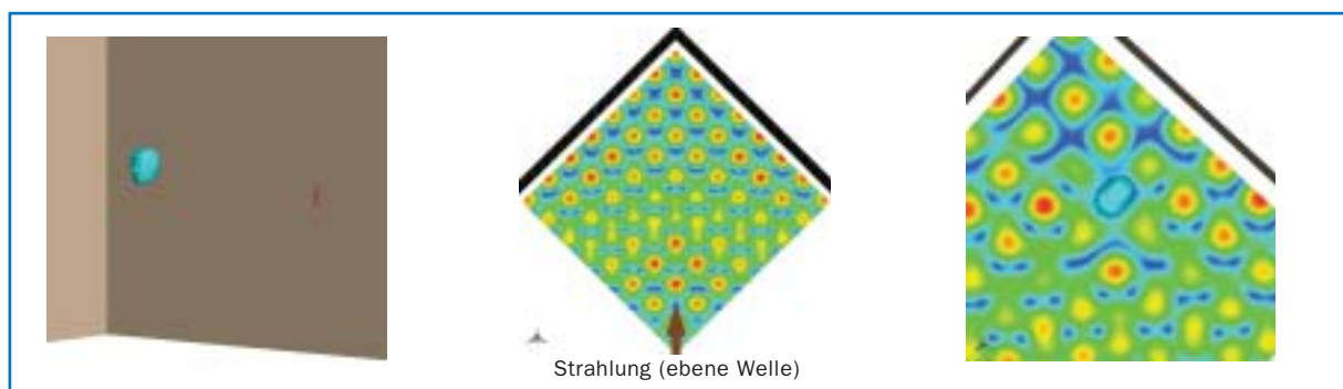
Bild 5: Ecke eines Zimmers, a) Ansicht, b) Interferenzfeld ohne und c) mit Kopf (Ausschnitt)
