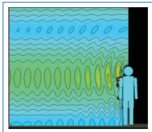
Bild 4: Feldstärkeverteilung vor einem Kind auf realem Boden
