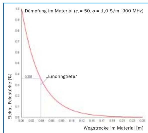
Bild 2: Eindringen einer Welle in ein verlustbehaftetes Medium
