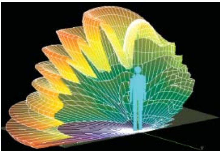
Bild 11: Richtungscharakteristik des ESM-140 bei 900 MHz über realem Boden. Man beachte die Interferenz zwischen reflektierter Bodenwelle und freier Raumwelle.
